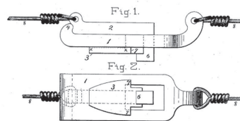
1890 Collegamento fusibile de-moltiplicato assemblato su un cavo (Frederick Grinnel's patent N°432403)
